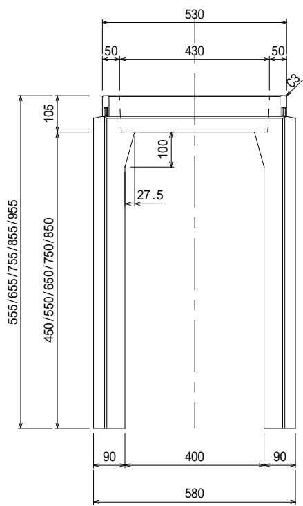
製品図 FW側溝A(凹凸部)400×400～800
