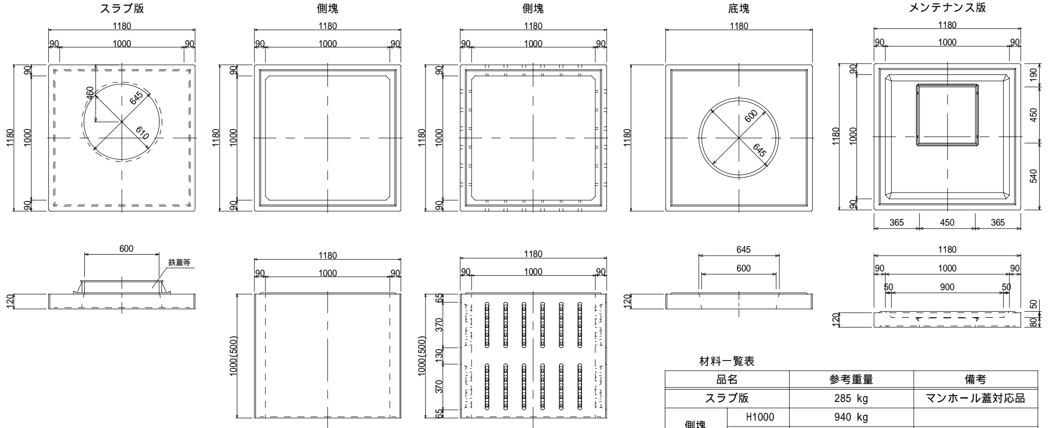
メンテナンス版組立断面図
