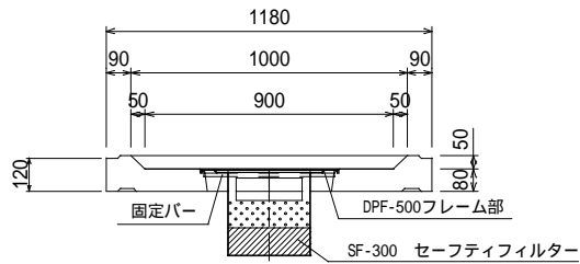
メンテナンス版組立断面図
