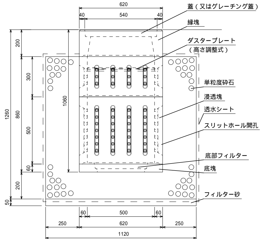
参考断面図（製品H=1060） ダスタープレート〔例〕
