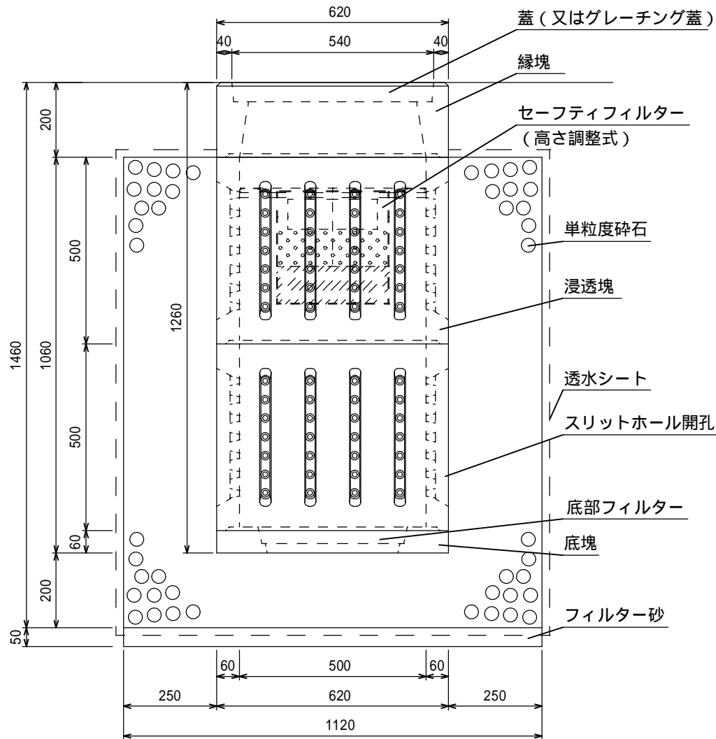
参考断面図（製品H=1260） セーフティフィルター〔例〕
