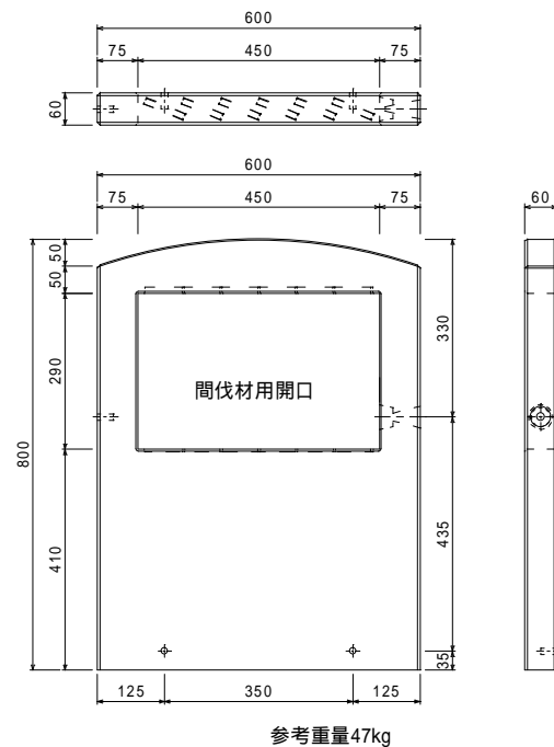
STW-0608R 600×H800 (天端R)
