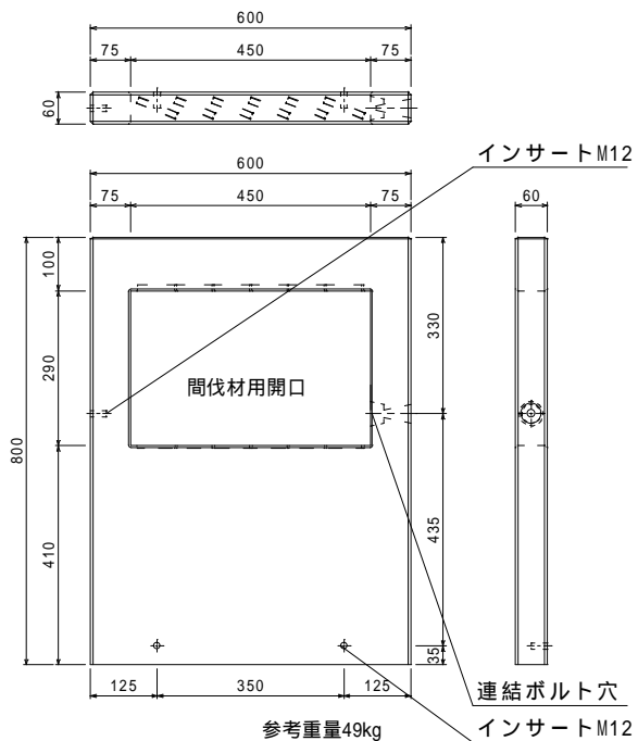
STW-0608F 600×H800 (天端フラット)
