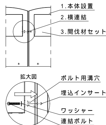
横連結方法
