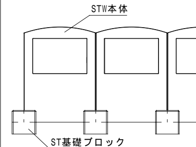
ST基礎ブロック使用例
